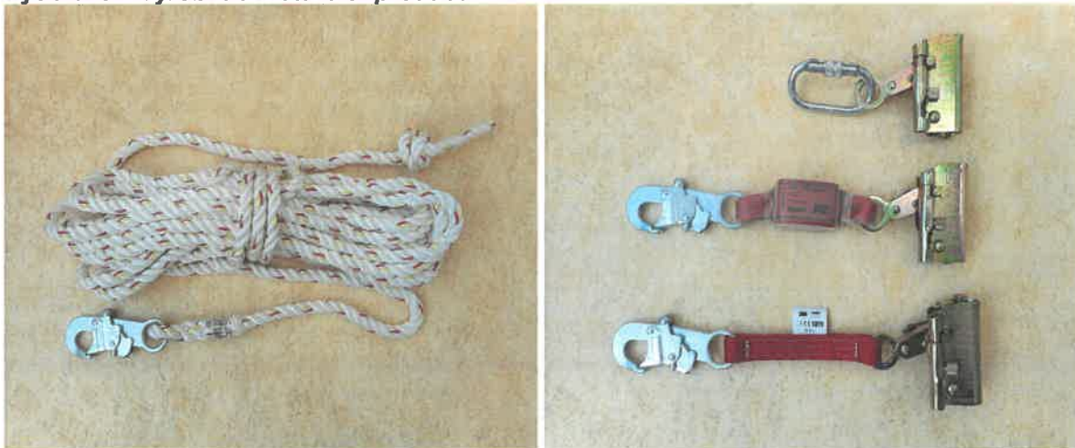
Záchytné zařízení vedeného typu na pružném kotvicím vedení Cobra, typ 5009017 a typ 5009004, 5009005, 5009006 Guided type all arrester including a flexible anchor line Cobra, type 5009017 and type 5009004, 5009005, 5009006
